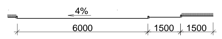
РОЗРІЗ 1-1
